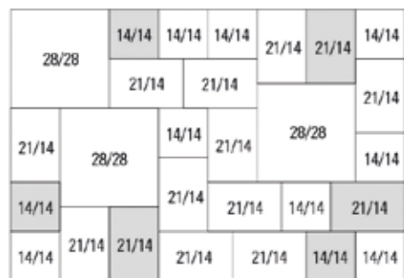
Rustikal Pflaster Mix Wilder Verband
